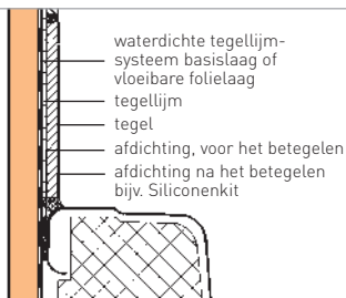
Afbeelding 27: Wandaansluitingen van douche of ligbaden (verticale doorsnede). Aansluiting aan FERMACELL enkel beplaatte montagewand bijvoorbeeld 1 S 11
