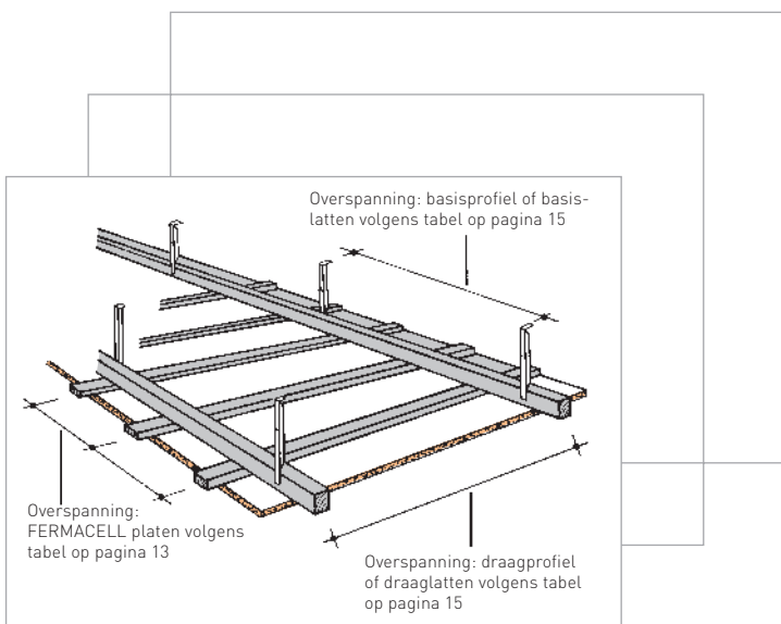
Afbeelding 9: Voorbeelden van houten latten en afhangers (metalene profielen of dezelfde wijze)
